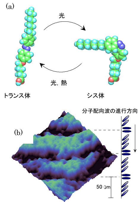
図 1 1. アゾベンゼン誘導体の光異性化反応 (a) と、それにより 2次元液晶に誘起される分子配向の伝播波。
